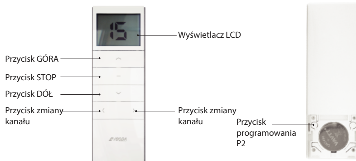
Nadajnik piętnastokanałowy
